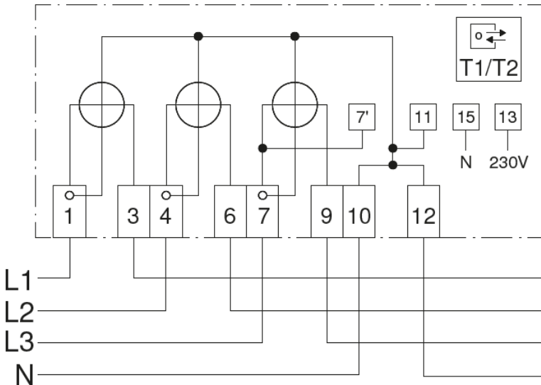
Abb. oben: Anschlussschaltbild 4102 (mit Zusatzklemmen, mit Tarifschaltklemmen)
