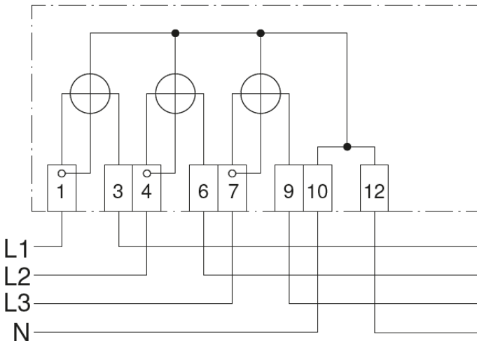
Abb. oben: Anschlussschaltbild 4000 (ohne Zusatzklemmen, ohne Tarifschaltung)
