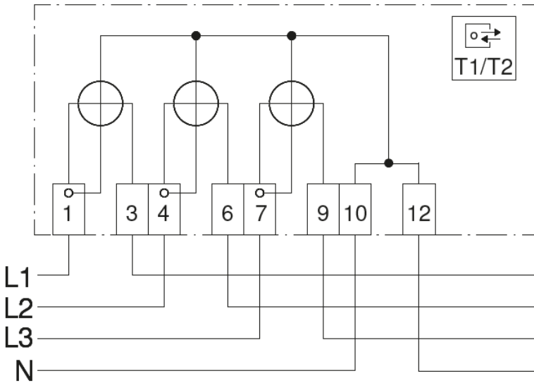
Abb. oben: Anschlussschaltbild 4100 (ohne Zusatzklemmen, ohne Tarifschaltklemmen, mit Tarifschaltung per SML über MSB-DSS)
